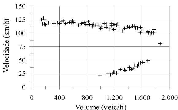
Figura 2: Variação da velocidade média com o volume de tráfego
